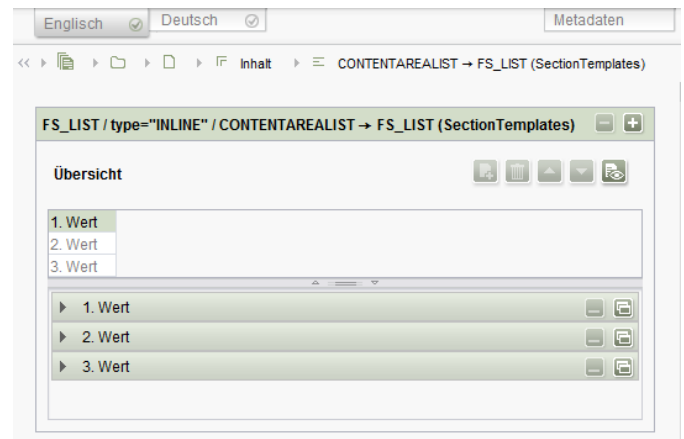
Eingabekomponente FS_LIST
