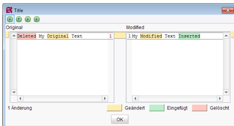
Vergleich ( OpenComparisonDialogOperation )
